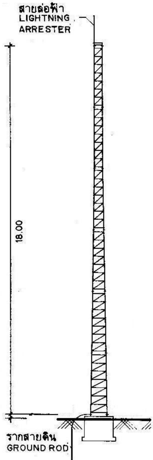
เสาโครงถักลอยตัว 18.00M. SELF-SUPPORT TOWER
