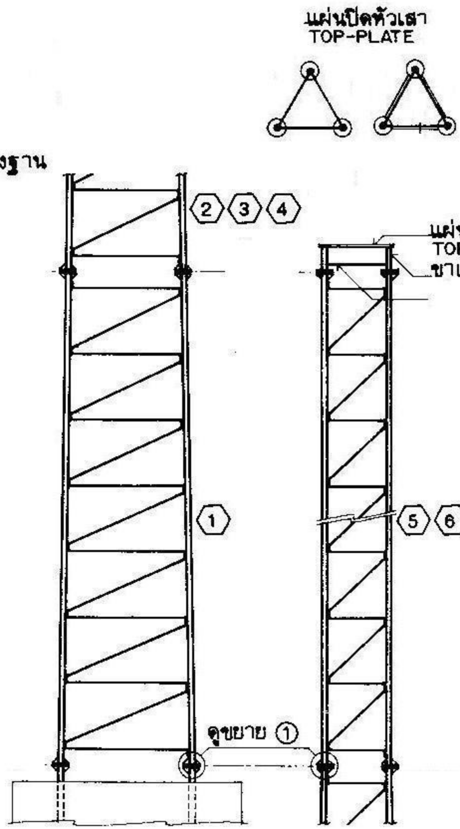
แบบขยายเสา TOWER DETAIL
