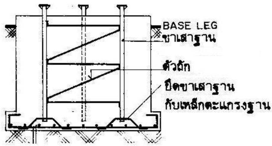
แบบขยายฐานเสา FOOTING DETAIL
